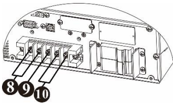
Diagramm 2: Eingangs-/Ausgangsklemme
