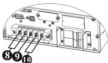
Diagram 2: Wejścia/Wyjścia Terminalu
